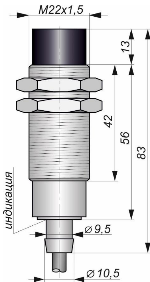
Габаритный чертеж
